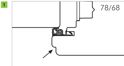
Zierprofilierung am Flügelüberschlag
