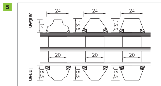
Sprossen – 3 Falzarten: Zierfalz, Schrägfalz*, Trapezfalz
