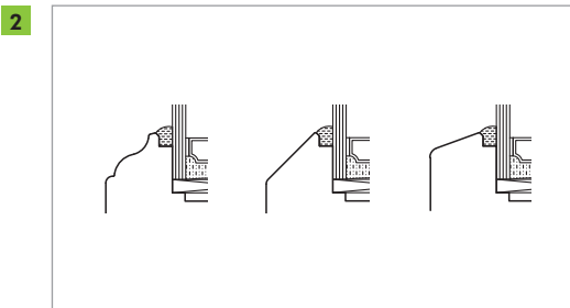
3 Falzarten: Zierfalz, Schrägfalz*, Trapezfalz
