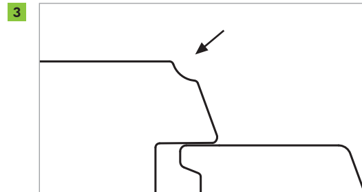
Einsetzfräsung im Rahmen
